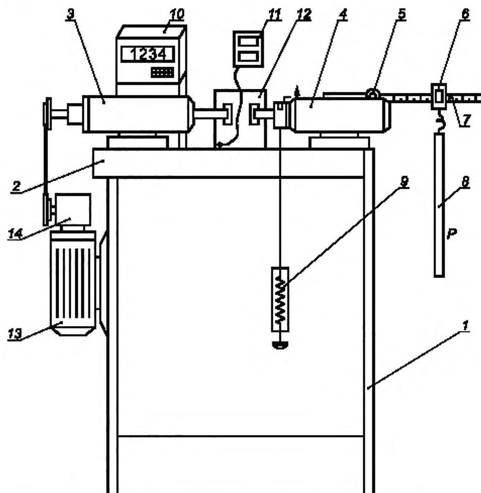
1 — станина; 2 — суппорт; 3 — неподвижная бабка; 4 — подвижная бабка; 5 — нажимное устройство; 6 — рамка (каретка); 7 — рейка кармывала; 8 — груз; 9 — динамометр; 10 — цифровой преобразователь; 11 — термометр; 12 — ювета для воды; 13 — электродвигатель; 14 — редуктор
