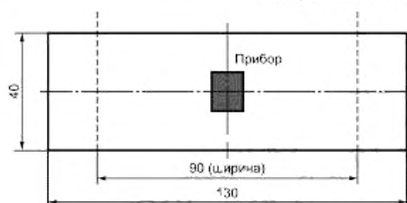
Рисунок 3 — Пример монтажа поверхностно монтируемого прибора для проведения испытаний на устойчивость при монотонном и циклическом изгибах
