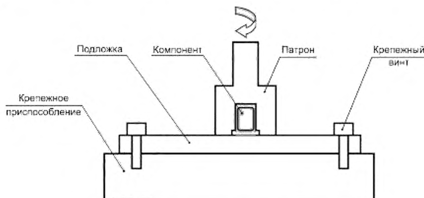
Рисунок 10 — Испытание на прочность при приложении крутящего момента
