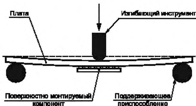
Рисунок D.1 — Пример приспособления для изгиба платы
