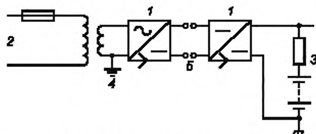
б) Зарядка аккумулятора постоянным током
