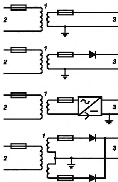
1 — разделительный трансформатор; 2 — первичный источник электроэнергии; 3 — цепь управления
