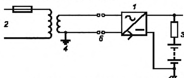
а) Зарядка аккумулятора переменным током
