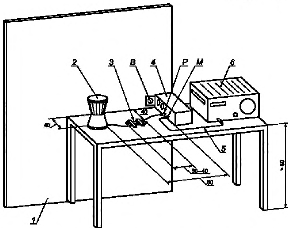
1 — металлическая стена 2 × 2 м; 2 — испытуемое ТС; 3 — излишек сетевого шнура, уложенный плоскими петлями 3 × 40 см; 4 — V-образный эквивалент сети; 5 — коаксиальная кабель; 6 — измерительный приемник; B — соединение с опорным заземлением; M — вход измерительного приемника; P — питание испытуемого ТС
