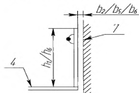
б) Ограничение доступа к краям платформы: предохранительный барьер (заслонка) и съемные ограждения для платформ с перемещением от 500 до 2000 мм
