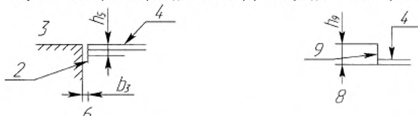
а) Вход на верхнюю или промежуточную посадочную площадку, фартук
