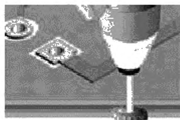
Рисунок 11 б — Фрезерование канавки в кромке печатной платы
