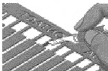
Рисунок 35 b — Удаление клеевой пленки с участка под паяное соединение
