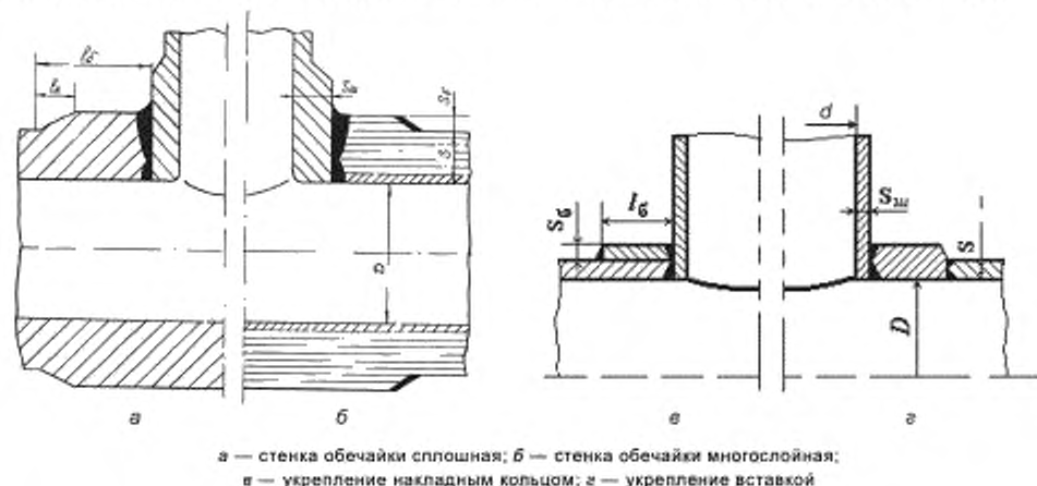
Рисунок 4.1 — Способы укрепления отверстий в обечайке (днище)
