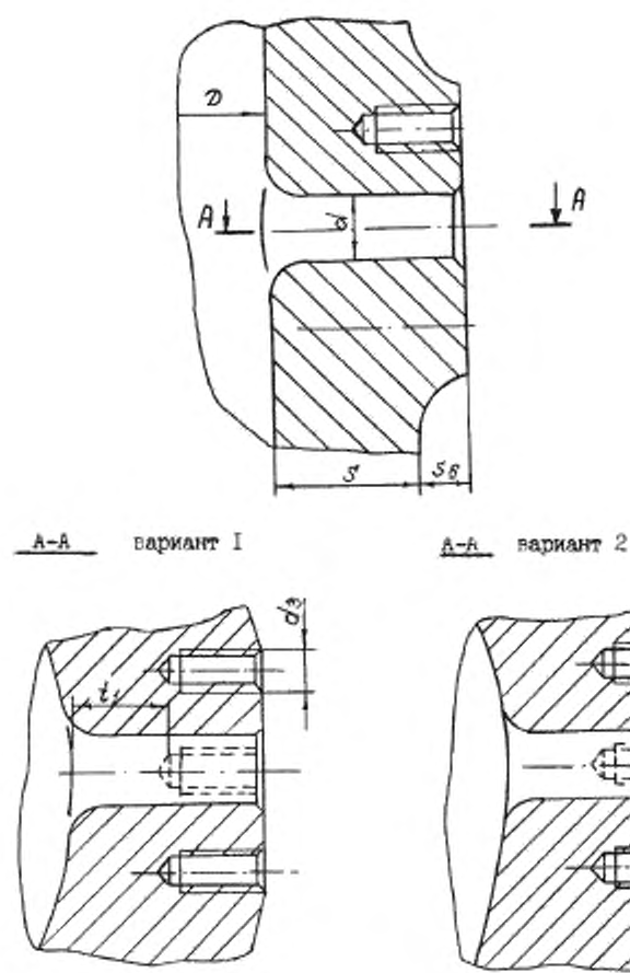
Рисунок 4.4 — Размещение резьбовых гнезд для крепежных элементов
