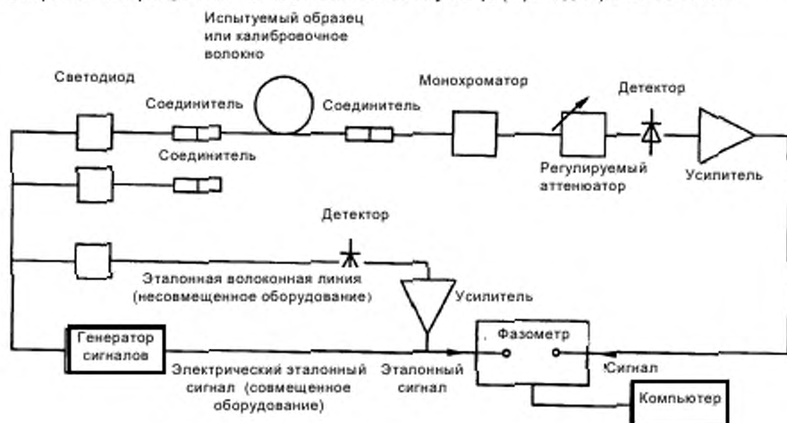
Рисунок A.3 – Комплект оборудования для измерения хроматической дисперсии. Система на основе светодиодов (типичная)
