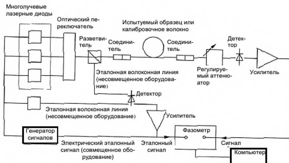
Рисунок А.1 – Комплект оборудования для измерения хроматической дисперсии. Система на основе многолучевого лазера (типовая)
