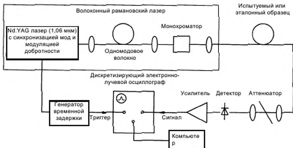
Рисунок В.1 – Структурная схема. Система на основе волоконного рамановского лазера
