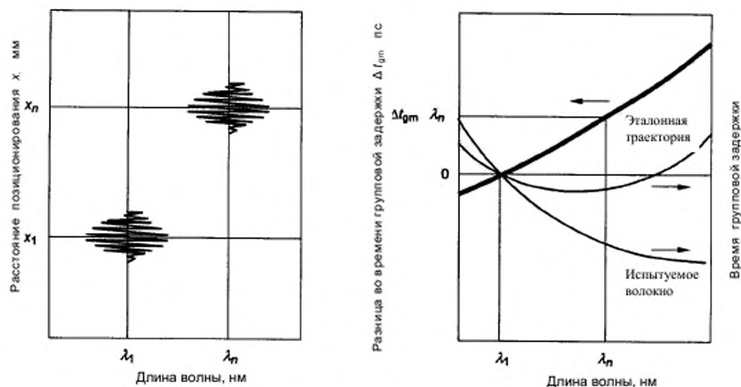
Рисунок D.3 – Примеры данных задержки
