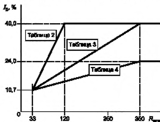
Рисунок А.1 — Зависимость норм гармонической составляющей тока 5-го порядка от R_{scc}
