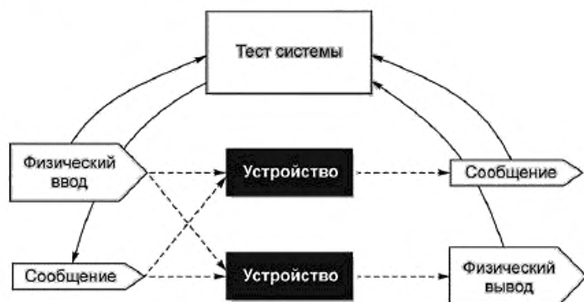
Рисунок 5 — Тестирование производительности (принцип черного квадрата)
