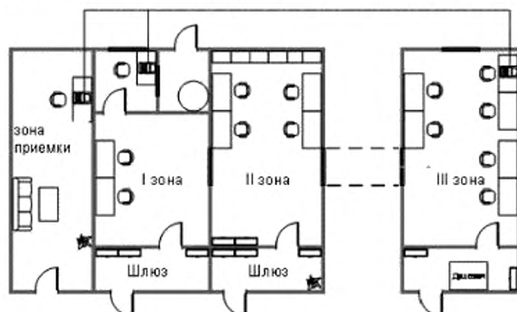
Рисунок А.1 — Схема ПЦР-лаборатории
