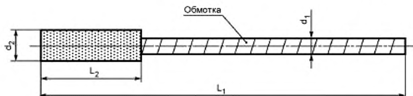
Рисунок Л.2 — Композитная гибкая связь с цилиндрическим песчаным анкерным участком
