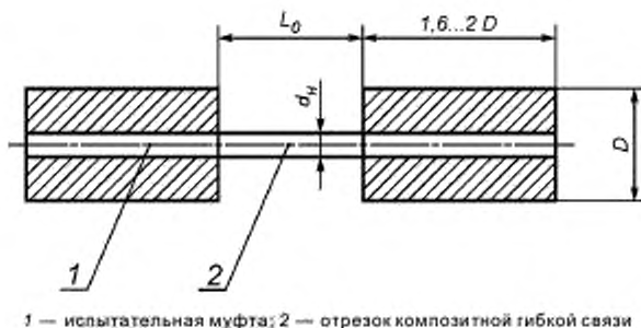
Рисунок В.2 — Общий вид образцов для испытания
