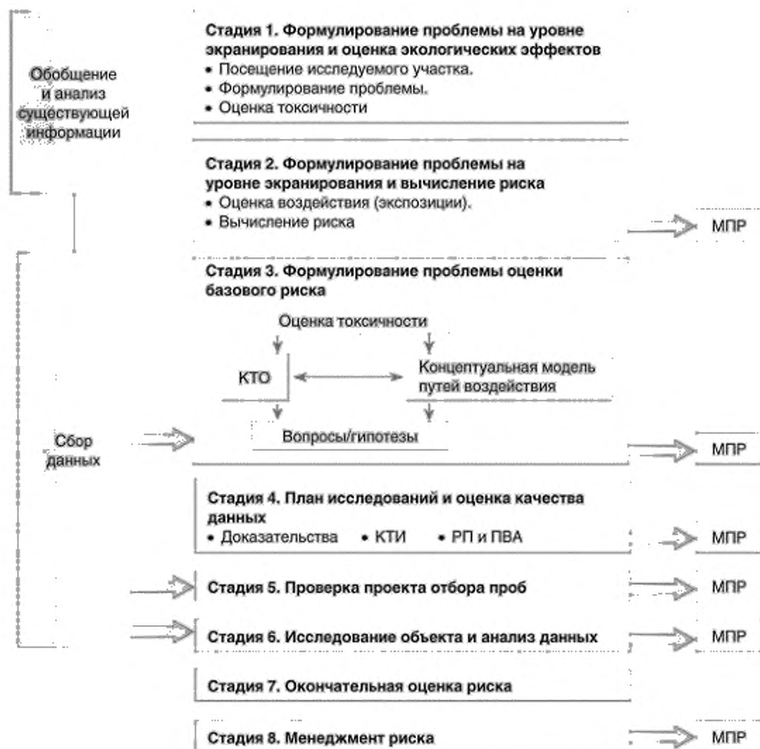
Рисунок 4 — Итеративный процесс общей оценки и снижения риска (МПР – момент принятия решения)
