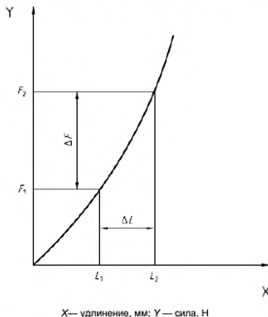
Рисунок 1 — Зависимость удлинения от силы при испытании на растяжение
