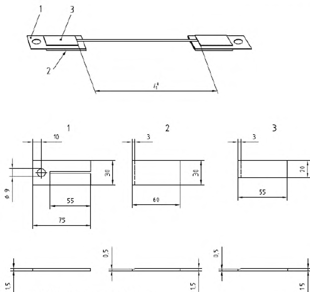
Рисунок С.4 — Петли из металлического листа
