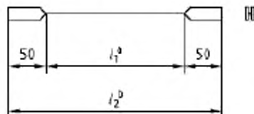
Рисунок С.2 — Петли из термореактивной смолы
