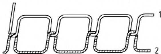
1 – игольная нитка, 2 – шпульчатая нитка
