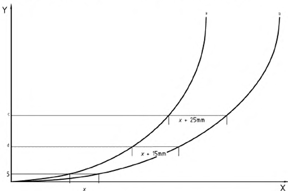
X – растяжение, мм; Y – сила, Н; a – несшитый образец; b – сшитый образец; c – нагрузка соответствующая открытию шва 5 мм; d – нагрузка, соответствующая открытию шва 3 мм
