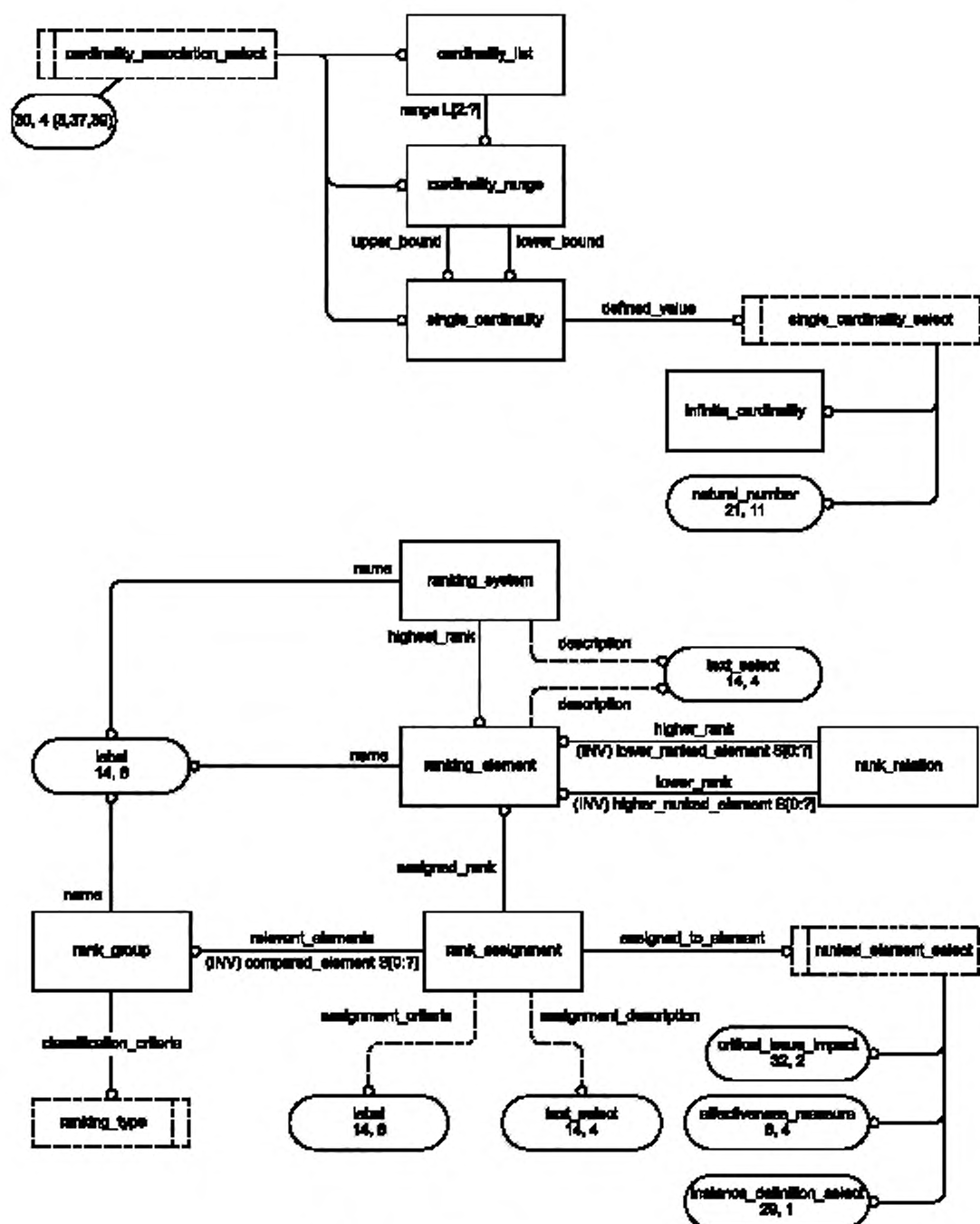
Рисунок E.31 — Диаграмма ссылочной модели приложения на уровне сущности в нотации EXPRESS-G (30 из 41)
