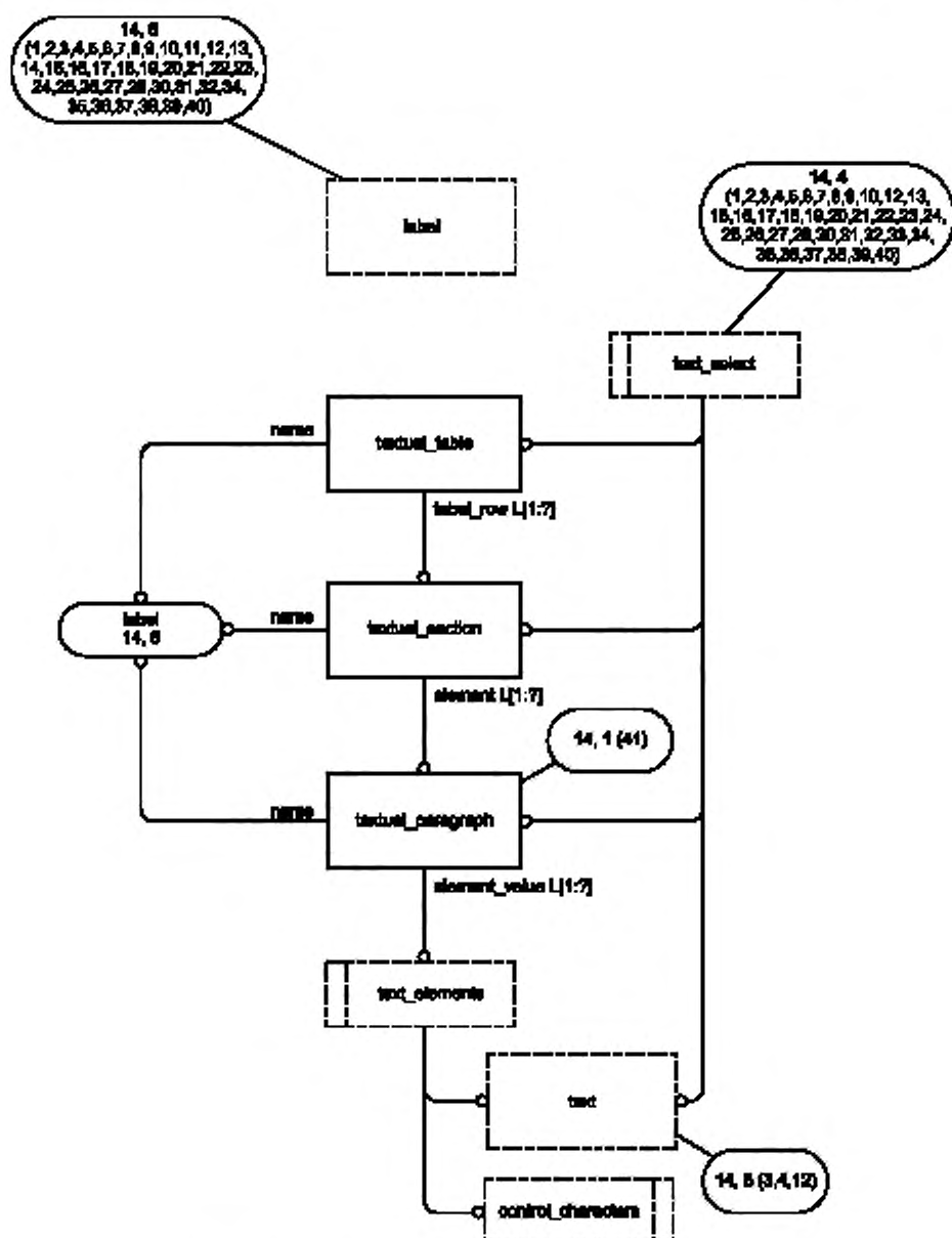
Рисунок E.15 — Диаграмма ссылочной модели приложения на уровне сущности в нотации EXPRESS-G (14 из 41)
