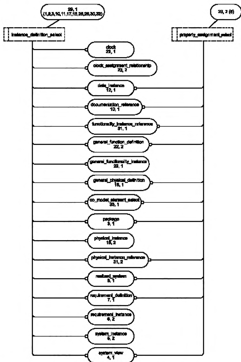
Рисунок E.30 — Диаграмма ссылочной модели приложения на уровне сущности в нотации EXPRESS-G (29 из 41)
