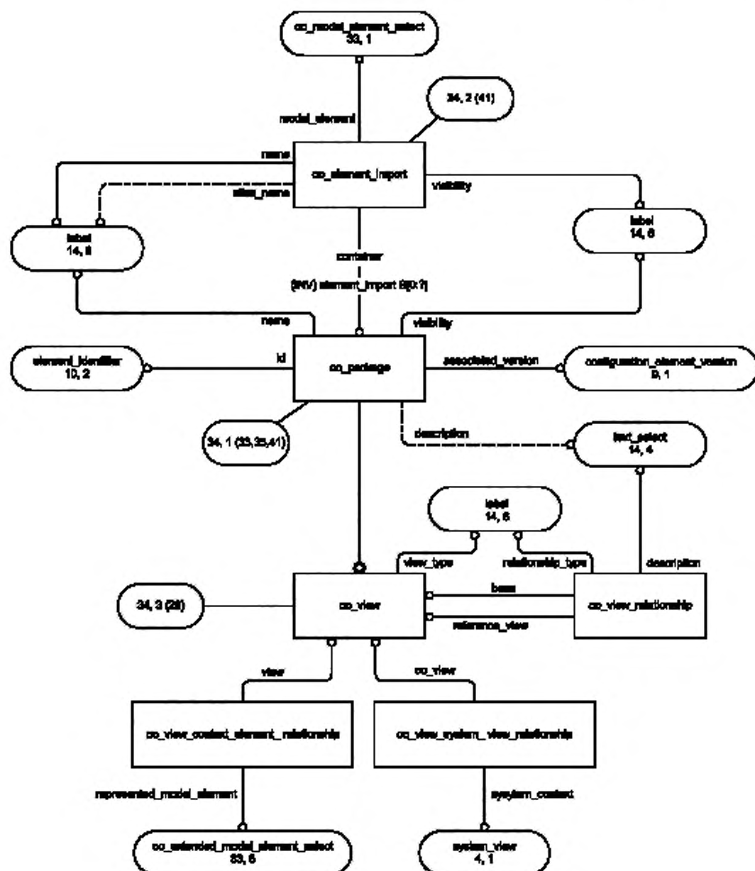
Рисунок E.35 — Диаграмма ссылочной модели приложения на уровне сущности в нотации EXPRESS-G (34 из 41)
