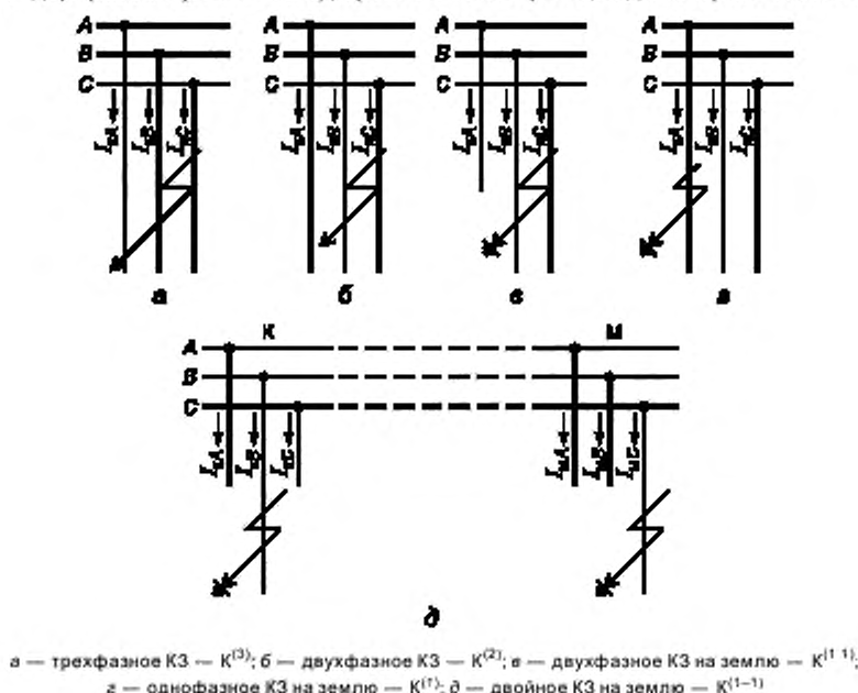
Рисунок 1 — Виды коротких замыканий
