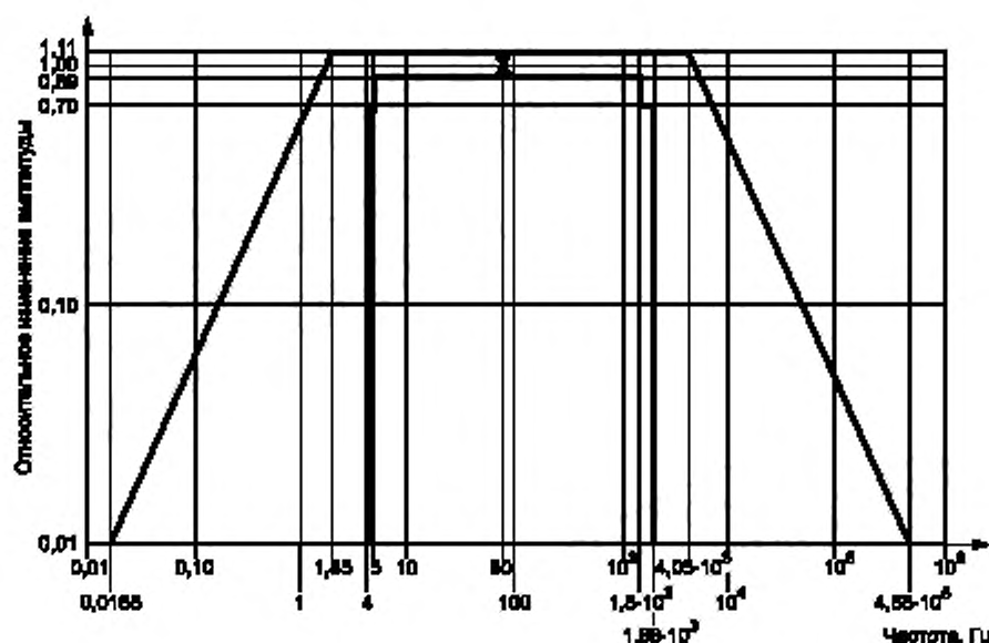
Рисунок 6 — Границы допусков для амплитудно-частотной характеристики
