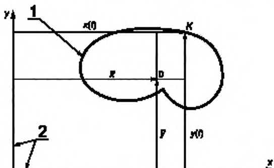
1 — траектория движения вала; 2 — координатные оси; O — среднее положение вала; K — мгновенное положение центра вала; x, y — средние значения перемещения вала; x(t), y(t) — мгновенные значения перемещения вала
