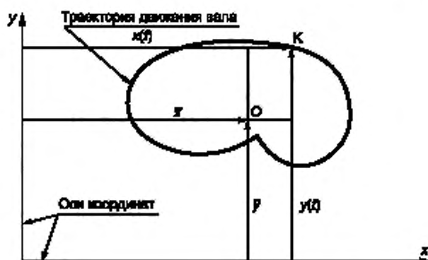
О — среднее положение траектории; К — мгновенное положение центра вала; \bar{x}, \bar{y} — среднее значение перемещения вала; x(t), y(t) — изменяющиеся со временем значения перемещения вала
