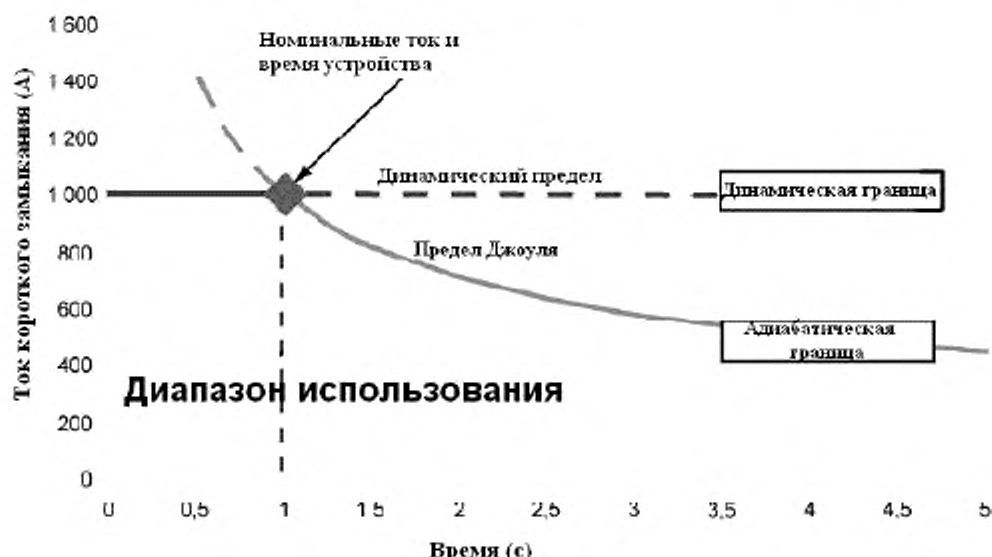
Рисунок С.4 – Пример используемого диапазона для устройства
