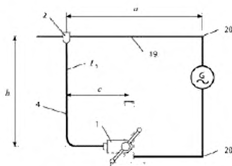
Рисунок 6f – Для испытуемых кабелей заземления согласно рисунку 3
