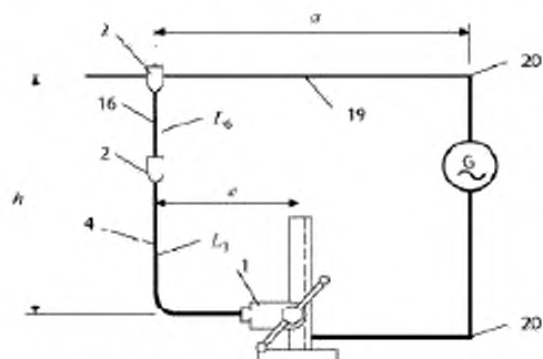
Рисунок 8b – Схема испытаний многополюсных устройств с токопородом для подвесных линий и для открытых подстанций в соответствии с рисунком 2g
