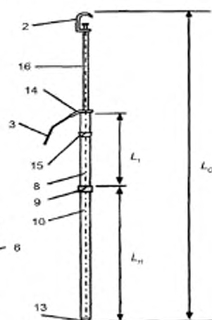
Рисунок 1б — Однополюсное оборудование с токопроводом
