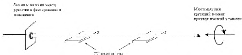
Рисунок В.2 – Схема испытаний на кручение на заземляющих стержнях с круглым поперечным сечением
