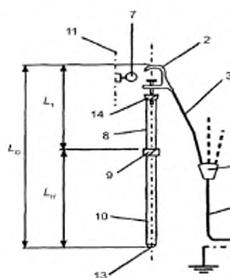
Рисунок 1а — Многополюсное оборудование
