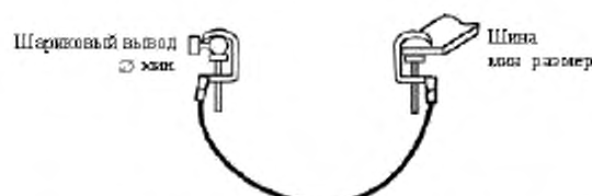
Рисунок 5д — Комбинация шарикового вывода и шины минимального размера
