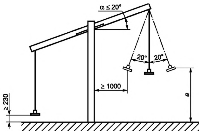
\alpha — максимальный угол отклонения перекладины; a — высота свободного падения
