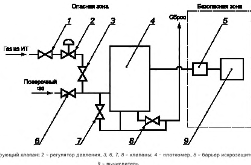
Рисунок 7 — Типовая схема монтажа потокового плотнотера для измерения плотности газа при стандартных условиях
