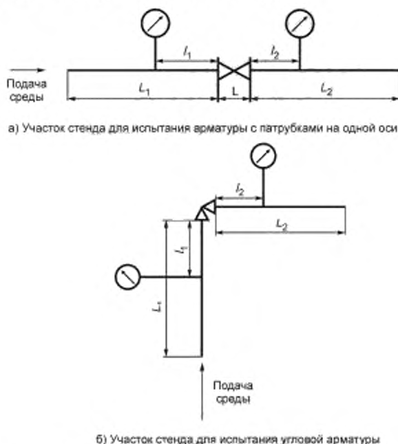
Рисунок 1 — Принципиальная схема испытательного участка гидравлического (пневматического) стенда
