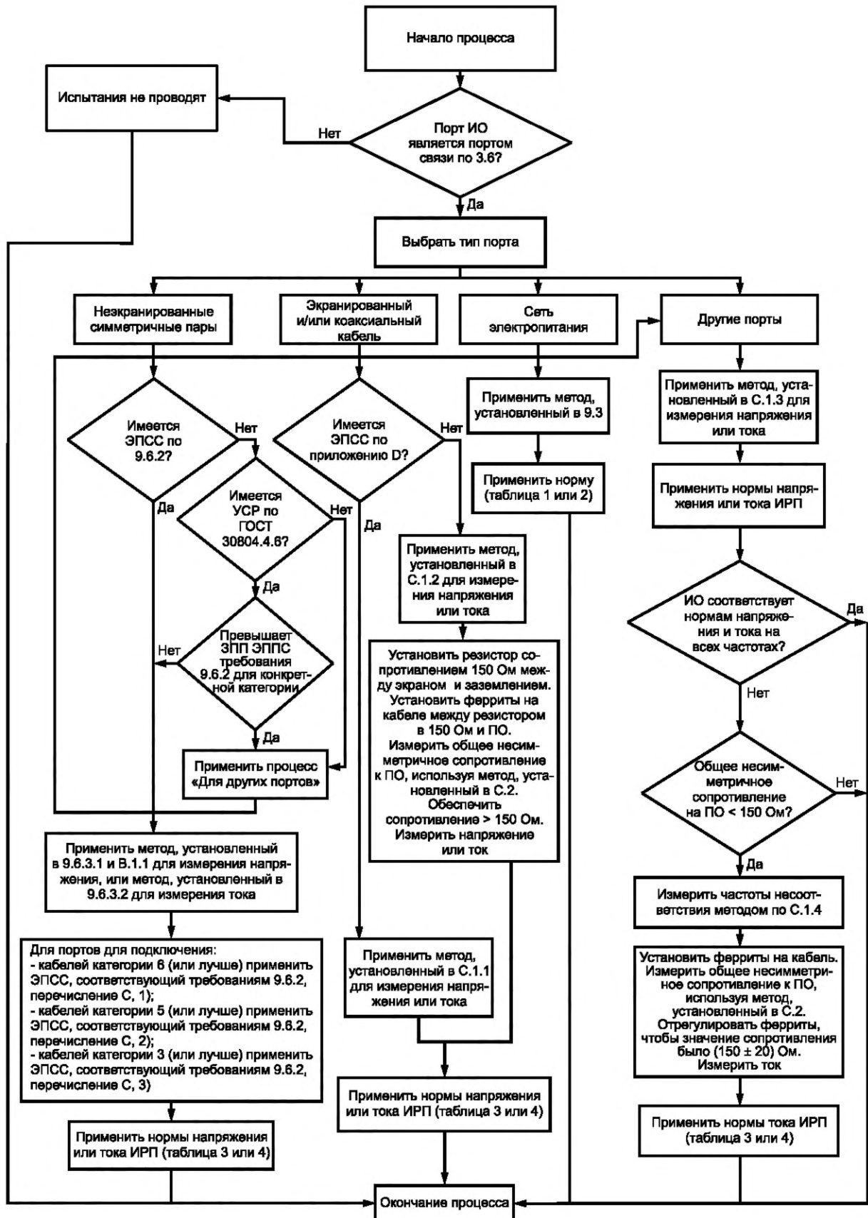
Рисунок С.6 — Алгоритм выбора методов испытаний
