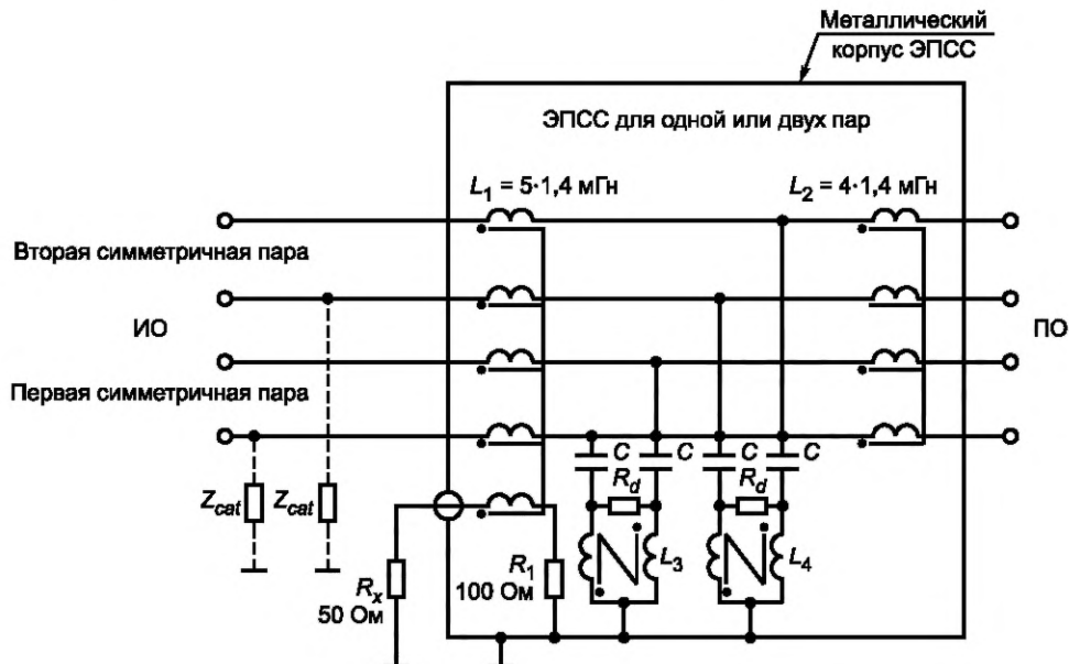
Рисунок D.1 — ЭПСС для применения с одной незранированной симметричной парой
