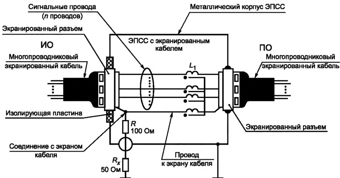
ПО — подключаемое оборудование; ИО — испытуемое оборудование; R_x — вход измерителя ИРП; дроссель общего несимметричного режима L_1 = (n + 1) \cdot 7 \text{ мГн} , где n — число сигнальных проводов
