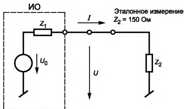
ИО — испытуемое оборудование; Z_1 — общее несимметричное полное сопротивление ИО; U_0 — напряжение источника ИРП; U — общее несимметричное напряжение ИРП на порте связи; I — общий несимметричный ток ИРП на порте связи; Z_2 — общее несимметричное полное сопротивление нагрузки
