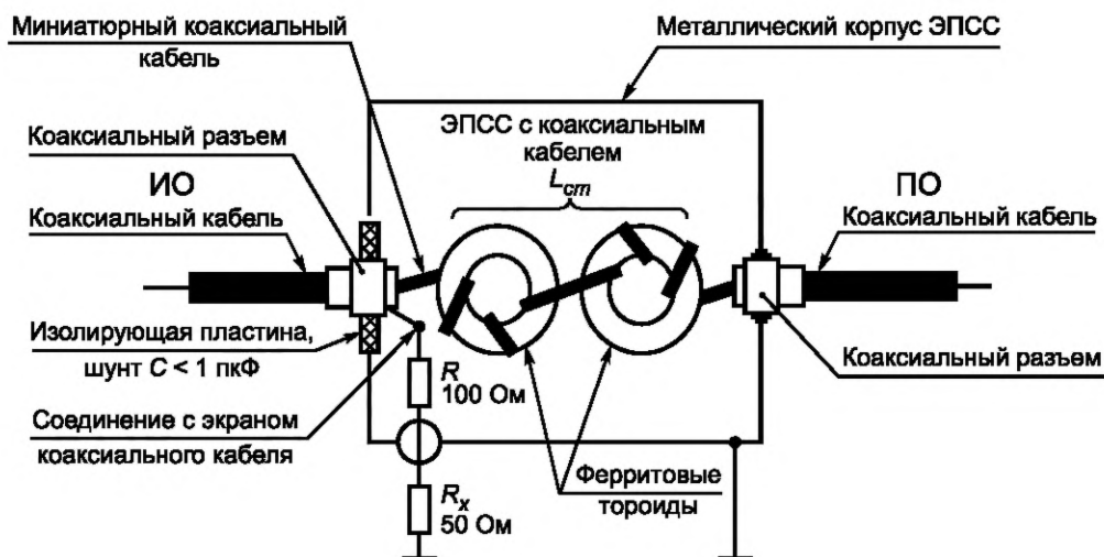
ПО — подключаемое оборудование; ИО — испытуемое оборудование; R_x — вход измерителя ИРП; дроссель общего несимметричного режима L_{cm} > 9 \text{ мГн} , паразитная емкость C < 1 \text{ пкФ}
