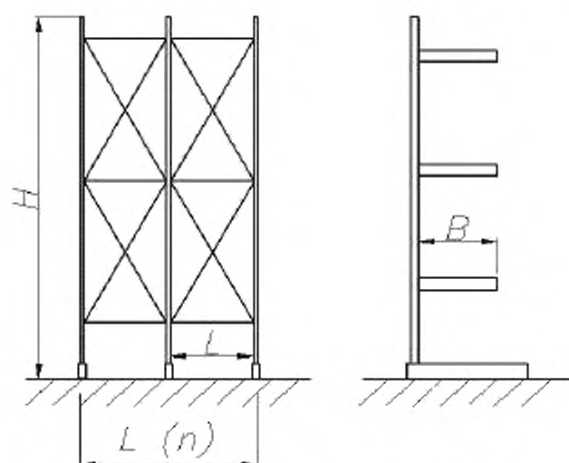
Рисунок 3 – Общий вид консольного стеллажа
