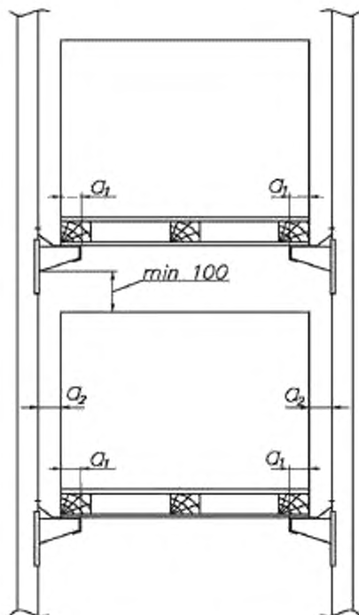
Рисунок 8 – Размещение груза относительно опорных профилей (грузонесущих направляющих)
