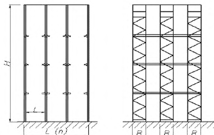
Рисунок 2 – Общий вид набивного (глубинного) стеллажа
