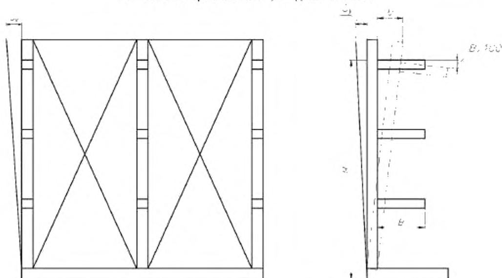
Рисунок 13 – Прогиб элементов консольных стеллажей
