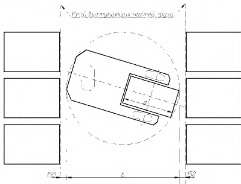
а – длина поддона с грузом; b – габариты ШТ с грузом на захвате Рисунок 4 – Параметры зазора между ШТ и грузами
