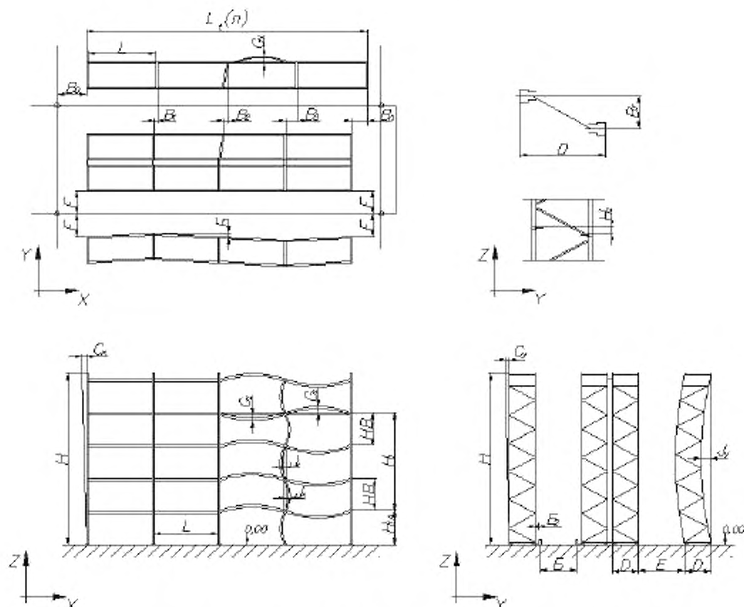
Рисунок 7 – Параметры, подлежащие контролю в ненагруженном состоянии системы
