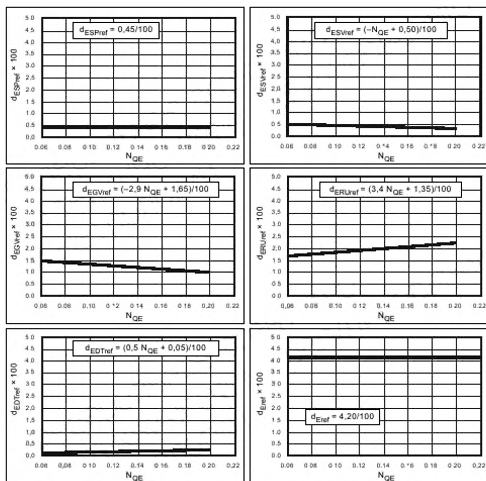
Рисунок В.12 — d_{ECOref} и d_{Eref} для турбопоса при работе в режиме насоса
