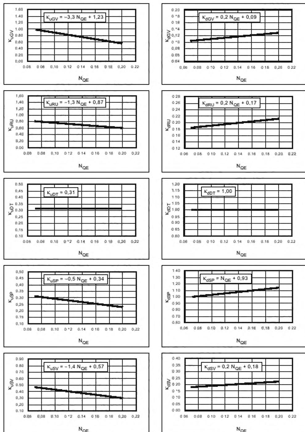
Рисунок В.8 — \kappa_{uCO} и \kappa_{dCO} для каждого компонента турбонасоса при работе в режиме турбины
