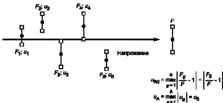
Рисунок 3 — Бюджет составляющих неопределенности при калибровке (пример для 5 уровней напряжения)
