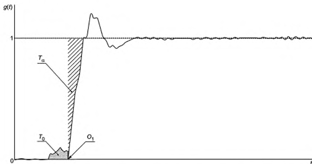
Рисунок В.2 — Нормализованная переходная характеристика g(t) , демонстрирующая начальное искажение начального времени искажения T_0
