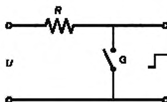
Рисунок В.3.д — Типовая схема цепи ступенчатого генератора
