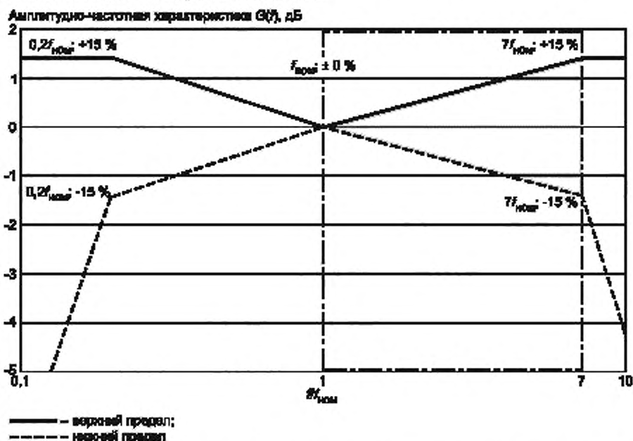
Рисунок 6 — Приемлемая нормализованная амплитудно-частотная характеристика измерительной системы (затененная область), предназначенной для измерения одной из основных частот f_{\text{ном}} (испытанная в диапазоне 1-7f_{\text{ном}} )
