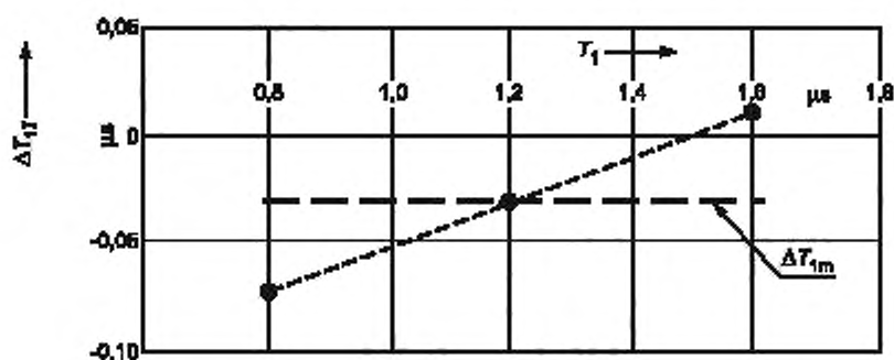
Рисунок Б.2 — Отклонение времени нарастания фронта (длительности переднего фронта) \Delta T_1 измерительной системы X по отношению к эталонной измерительной системе N и их среднее значение \Delta T_{1m} в диапазоне T_1 = 0,8 \dots 1,6 \text{ мкс}
