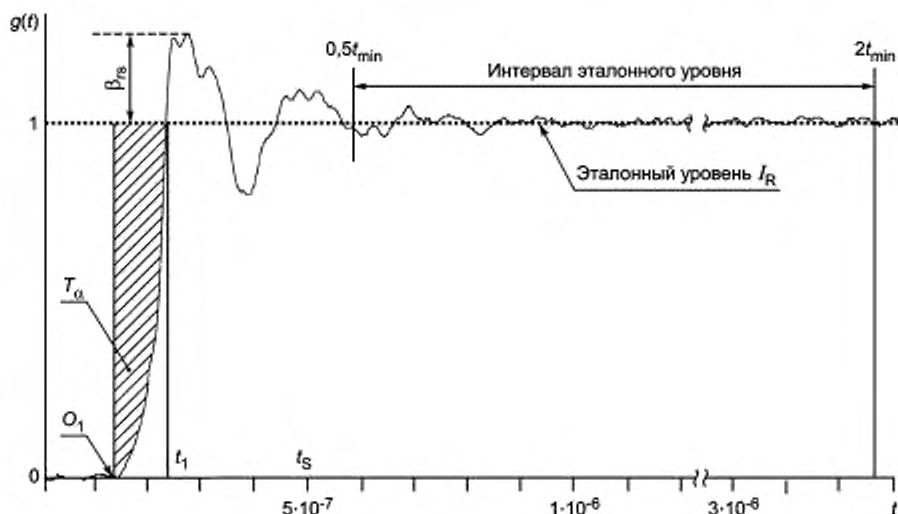
а — Определения для нормализованной переходной характеристики g(t)
