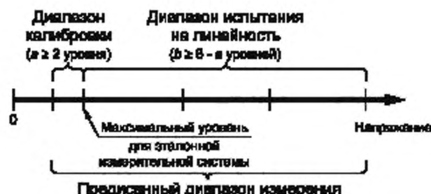
Рисунок 4 — Калибровка методом сличения с дополнительным испытанием на линейность
