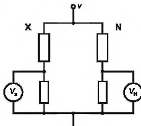
Рисунок Б.1 — Сличение испытываемой системы X с эталонной системой N
