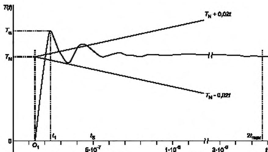
б — Определения интеграла переходной характеристики T(t)
