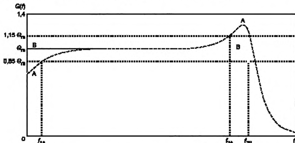
Рисунок 1 — Амплитудно-частотная характеристика с примерами предельных частот ( f_1 ; f_2 )
