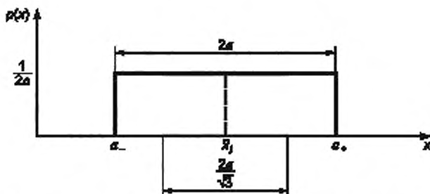
Рисунок А.2 — Плотность равномерного распределения вероятности p(x)
