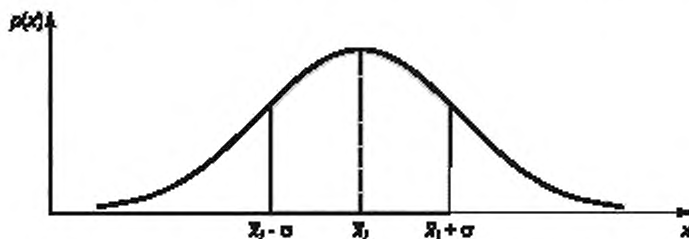
Рисунок А.1 — Плотность нормального распределения вероятности p(x)
