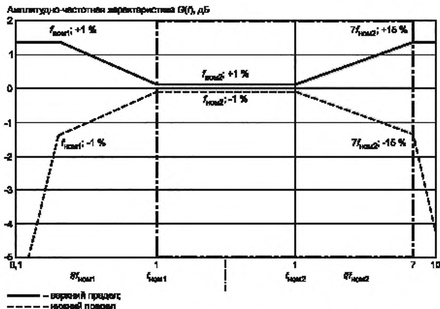
Рисунок 7 — Приемлемая нормализованная амплитудно-частотная характеристика измерительной системы (затененная область), предназначенная для диапазона основных частот от f_{\text{ном1}} до f_{\text{ном2}} (испытанная в диапазоне f_{\text{ном1}} - 7f_{\text{ном2}} )
