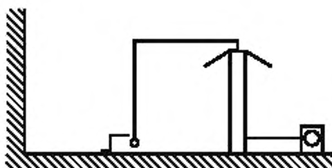
Рисунок В.3.б — Предпочтительная схема цепи для больших делителей
