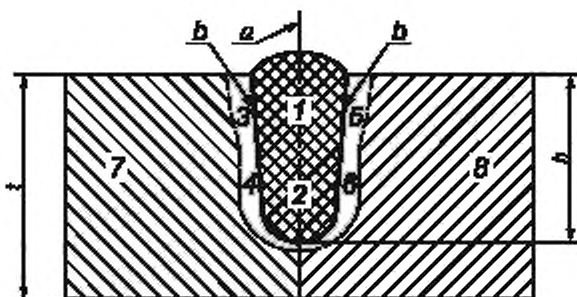
Обозначения: 1, 2 — металл сварного шва; 3, 4, 5, 6 — зоны термического влияния (HAZ); 7, 8 — основной металл, а — центр металла сварного шва; б — линия сплавления.
