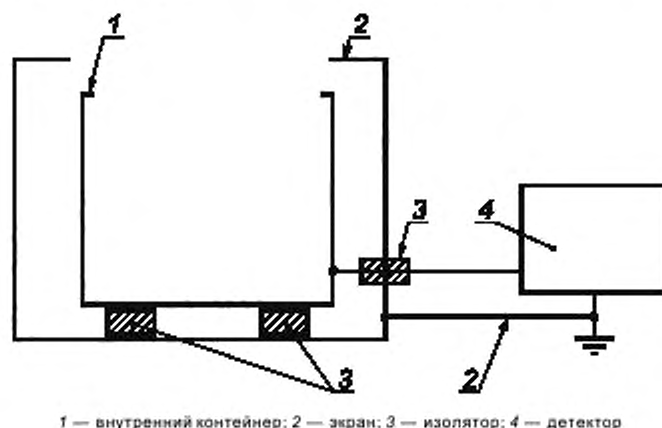
Рисунок 1 — Цилиндр Фарадея
