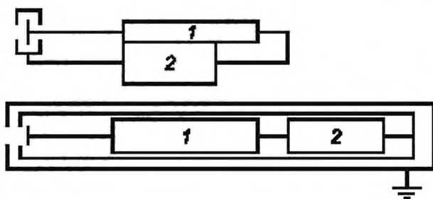
Рисунок 6 — Измеритель поля с обратной связью
