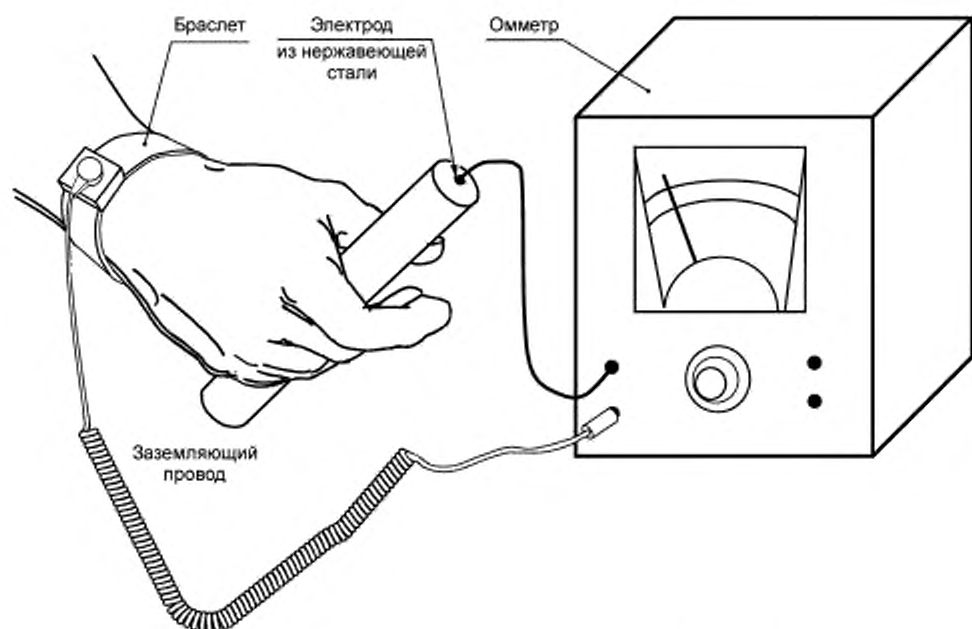
Рисунок 3 — Измерение сопротивления системы браслета
