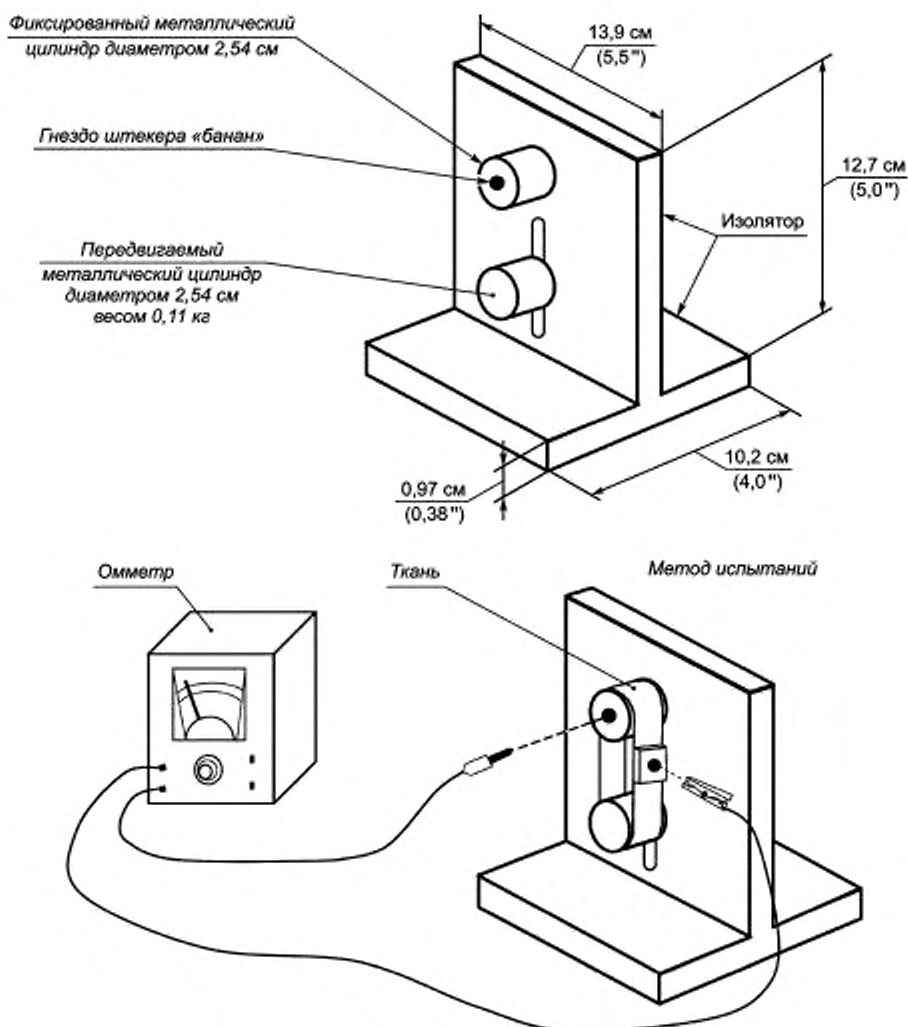
Рисунок 1 — Оборудование для измерения сопротивления браслета
