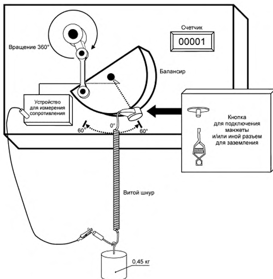
Рисунок 2 — Оборудование для измерения гибкости заземляющего провода
