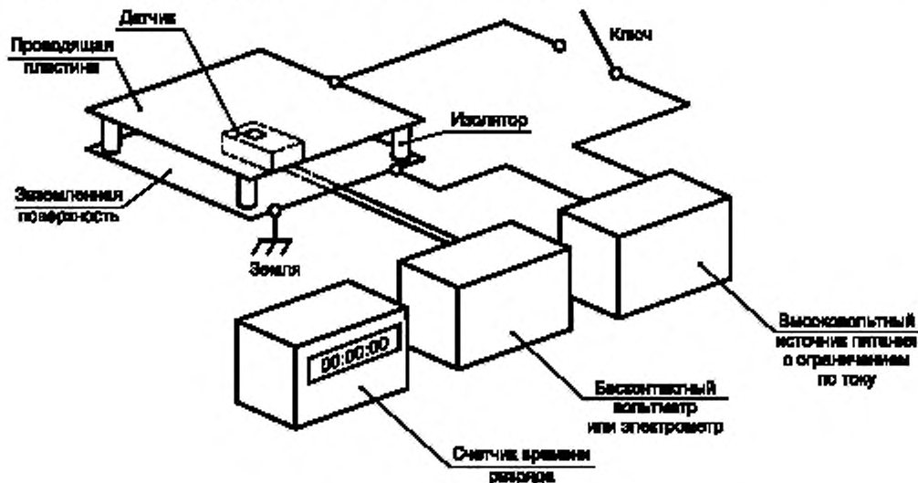
Рисунок 1 – Схема подключения измерительной пластины
