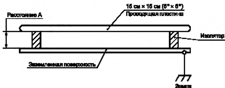
Рисунок 1 – Схема подключения измерительной пластины
