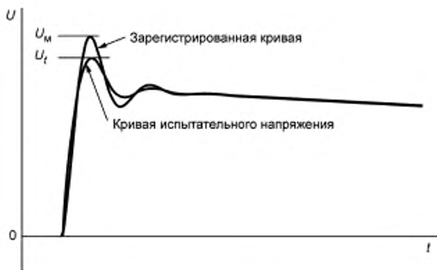
Рисунок Б.3 — Импульс испытательного и зарегистрированного напряжений
