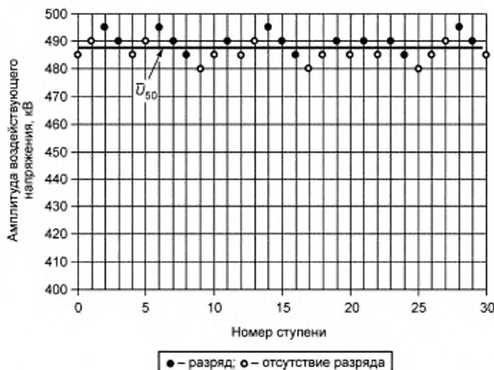
Рисунок А.3 — Результаты испытаний изоляции методом «вверх-вниз» (метод А.2.2)
