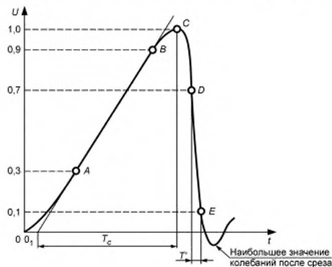
Рисунок 11 — Грозовой импульс, срезанный на фронте
