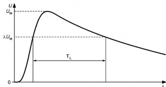
Рисунок 9 — Интервал времени импульсного напряжения
