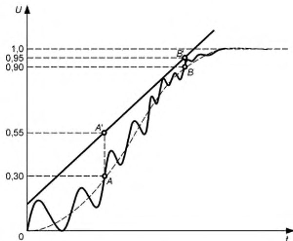
Рисунок 14 — Допустимые колебания на фронте импульса
