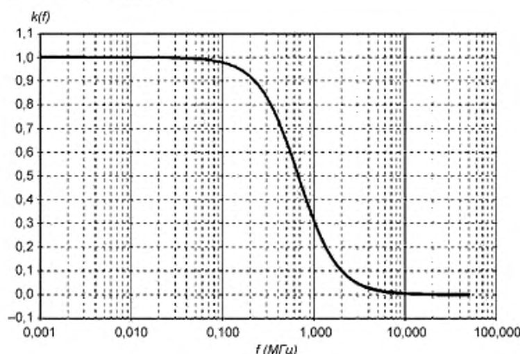
Рисунок 7 — Функция испытательного напряжения
