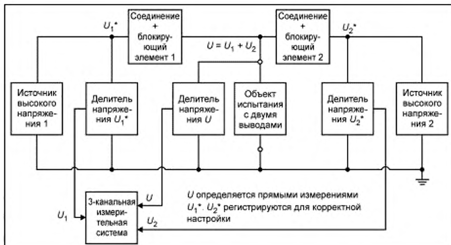
Рисунок 21 — Структурная схема испытаний наложенным напряжением
