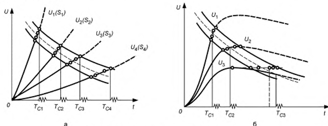
Рисунок 15 — Вольт-секундные характеристики изоляции
