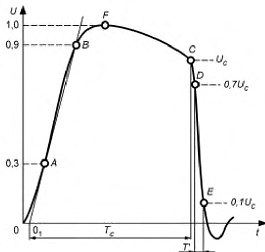
Рисунок 12 — Грозовой импульс, срезаемый на спаде импульса
