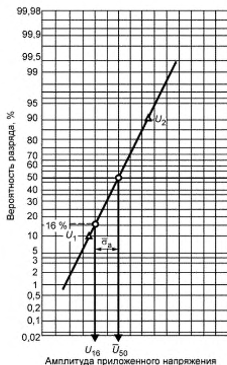
Рисунок А.2 — Кривая эффекта, построенная по результатам испытаний ступенчатым методом (А.2.1) по двум уровням напряжения
