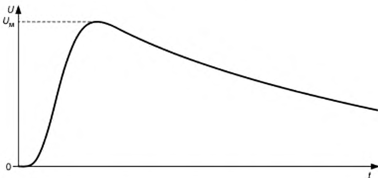
Рисунок 6 — Полный грозовой импульс напряжения
