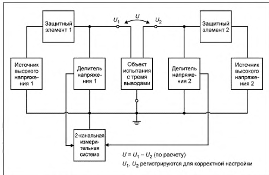
Рисунок 18 — Структурная схема испытаний комбинированным напряжением
