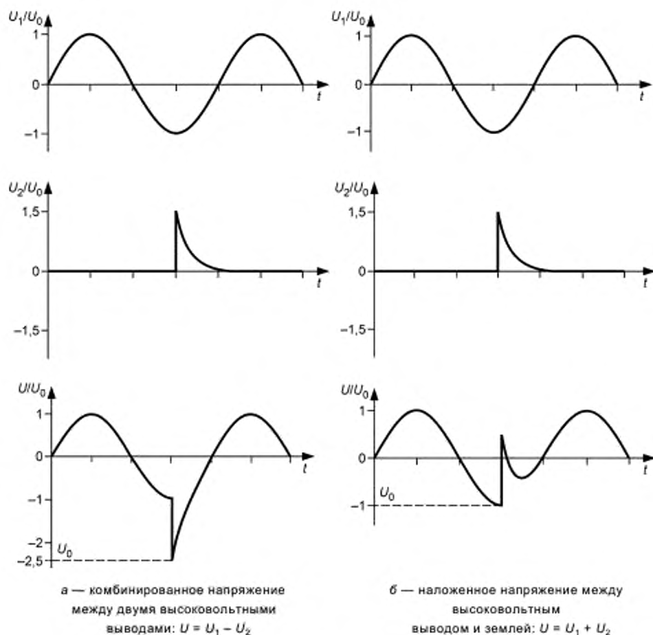
Рисунок 19 — Стилизованное представление комбинированного и наложенного напряжений
