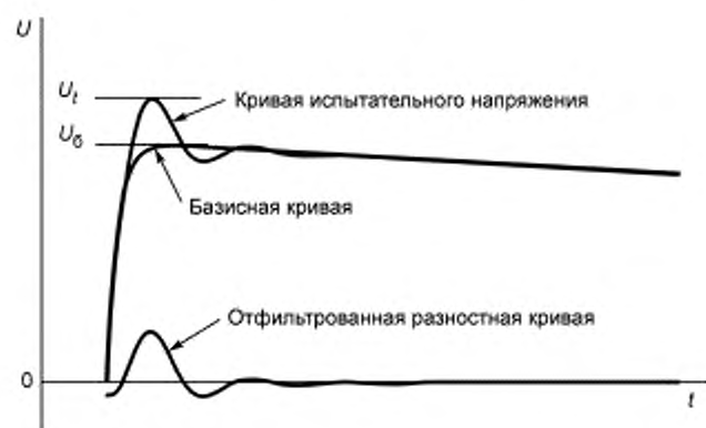
Рисунок Б.2 — Кривая испытательного напряжения, базисная кривая и отфильтрованная разностная кривая
