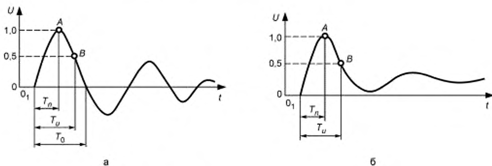
Рисунок 17 — Колебательный коммутационный импульс
