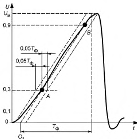
Рисунок 13 — Линейно нарастающий импульс, срезаемый на фронте
