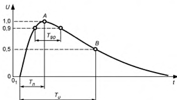
Рисунок 16 — Аperiodический коммутационный импульс
