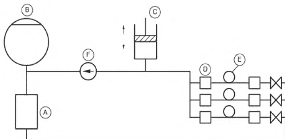
A — нагреватель с терморегулятором; B — напорный бак; C — генератор пульсаций; D — соединитель; E — шланг с петлей; F — насос
