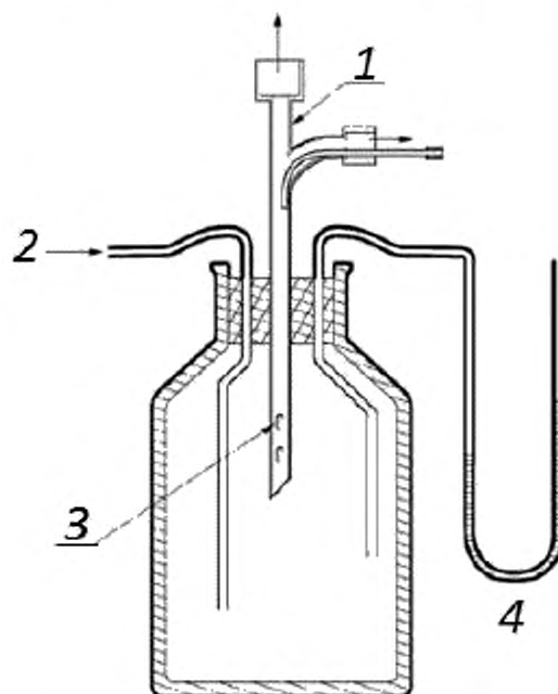
1 – жесткий бронхоскоп; 2 – поступление воздуха от средства измерений потока; 3 – боковые отверстия должны быть внутри резервуара; 4 – средство измерений давления, например, водяной манометр
