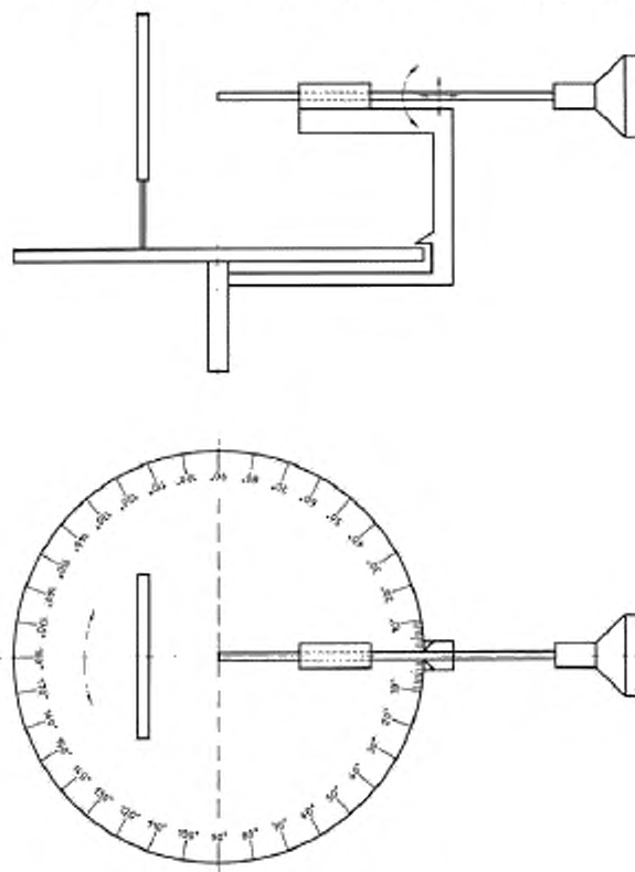
Рисунок 3 – Пример испытательной установки
