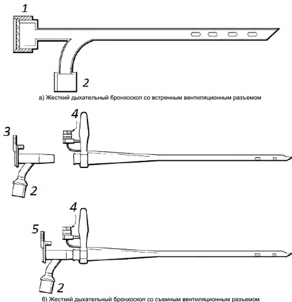
Рисунок 1 – Примеры жестких дыхательных бронхоскопов
