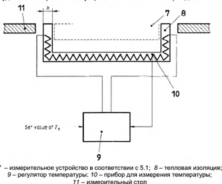
Рисунок 2 - Тепловая изоляция с регулятором температуры
