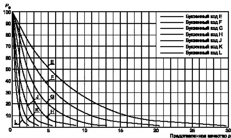
Рисунок 5 — Кривые ОС (PX) для планов однократного выборочного контроля, A_{SL}=0
