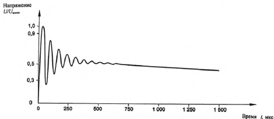
а) T_p / T_2 = 20 / 1\,000 мкс, 15 кГц
