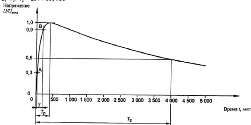
Рисунок 3 - Аперiodический коммутационный импульс
