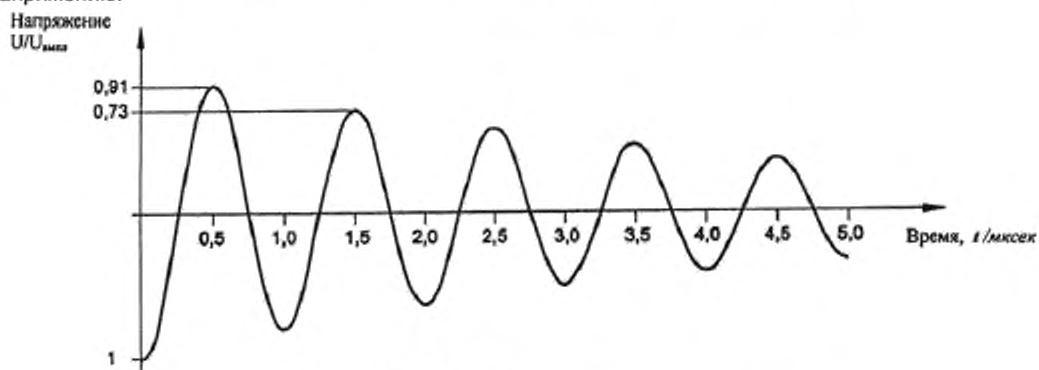
Рисунок 5 - Затухающее переменное напряжение
