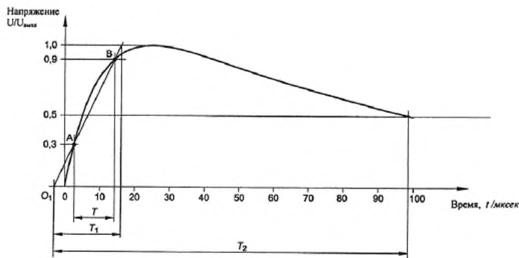
Рисунок 1 – Аперриодический грозовой импульс
