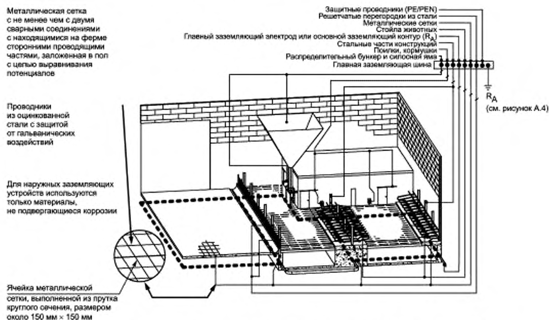
Рисунок А2 — Пример устройства выравнивания потенциалов, выполненного в виде кольца по периметру
