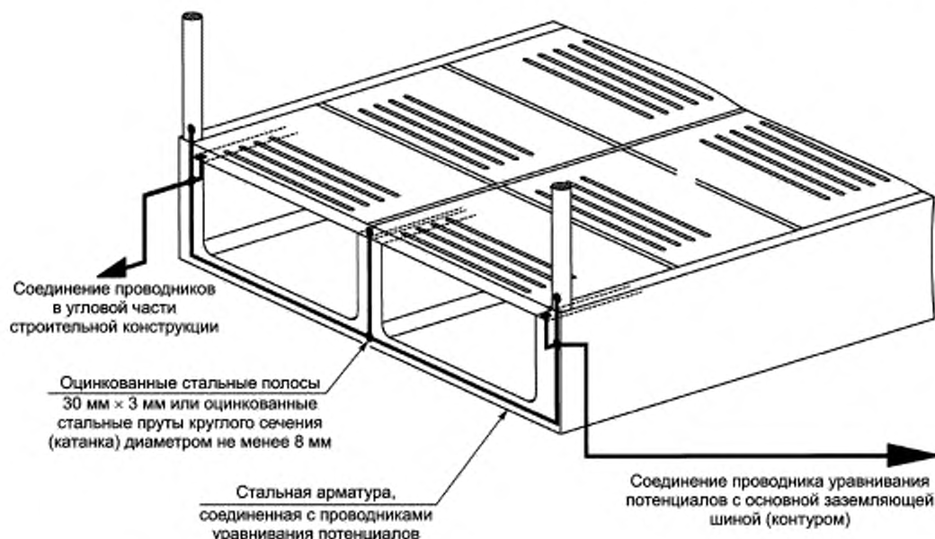
Рисунок А3 — Пример уравнивания потенциалов в бетонной строительной конструкции на этаже для сбора навоза
