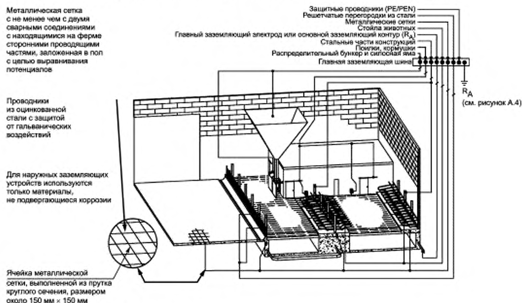
Рисунок А1 — Пример уравнивания потенциалов в коровнике
