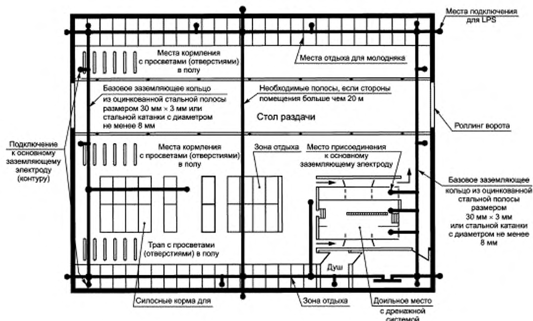
Рисунок А4 — Пример расположения основного заземляющего электрода в коровнике
