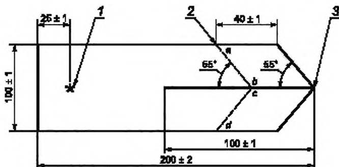
Рисунок 1 — Испытываемый образец в форме крыльев
