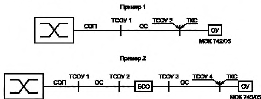
Рисунок 2 — Примеры сетевых конфигураций
