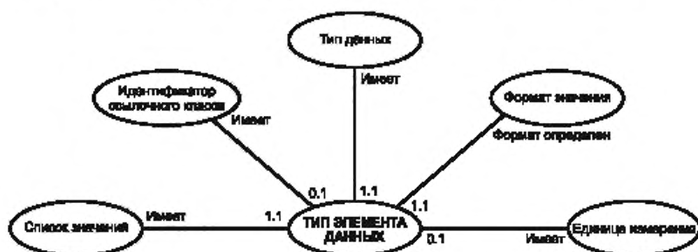
Рисунок 5 — Атрибуты значений типа элемента данных
