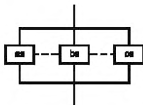
Рисунок А.5 — Иллюстрация объединенного защитного устройства
