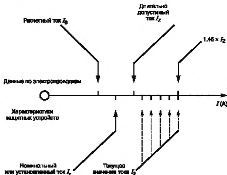
Рисунок В.1 — Иллюстрация условий 1 и 2 из 433.1
