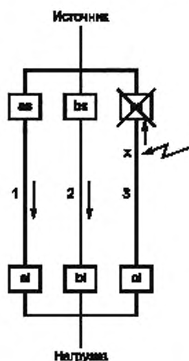
Рисунок А.4 — Электрический ток после срабатывания защитного устройства 'ca'
