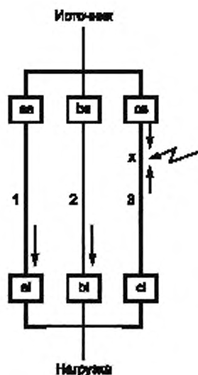
Рисунок А.3 — Электрический ток в начале отказа
