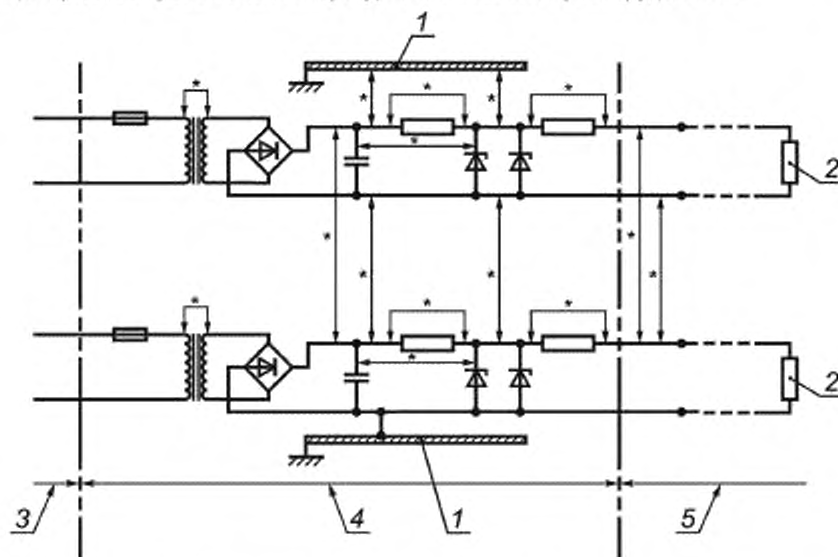
1 — шасси; 2 — нагрузка; 3 — взрывоопасная зона, заданная U_m ; 4 — часть искробезопасной цепи, не являющаяся искробезопасной; 5 — взрывоопасная зона; * — расстояния разделения, в отношении которых применяется таблица 4
