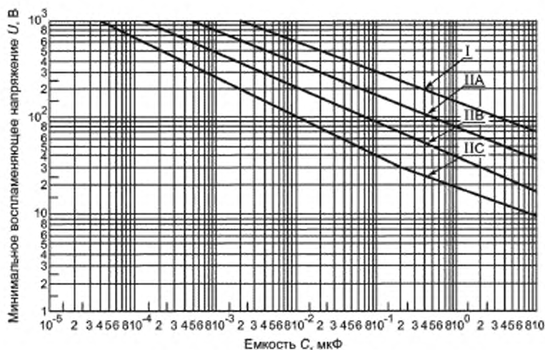
Рисунком A1.7 — Зависимость минимального воспламеняющего напряжения от емкости цепи
