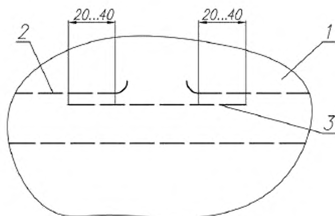
1 — ткань оболочки; 2 — разрушенная строчка, 3 — восстановленная строчка
