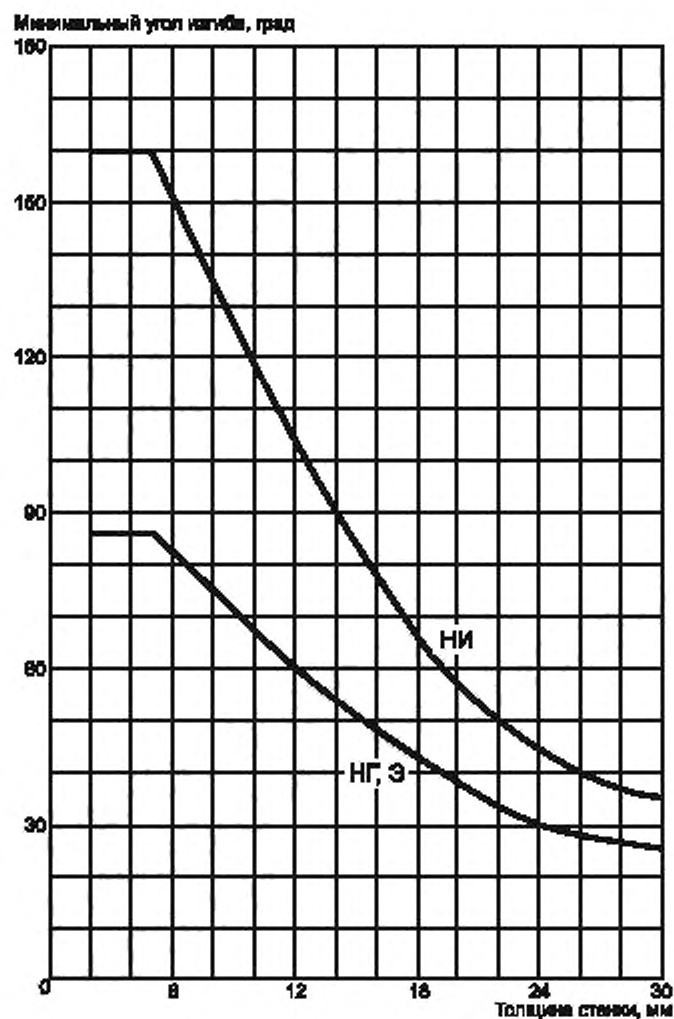
Рисунок В.3 — Минимальный угол изгиба для ПП-Р (тип 3) в зависимости от толщины для разных методов сварки (верхняя кривая — для сварки нагретым инструментом встык, нижняя — для пучковой газовой сварки и экструзионной сварки)
