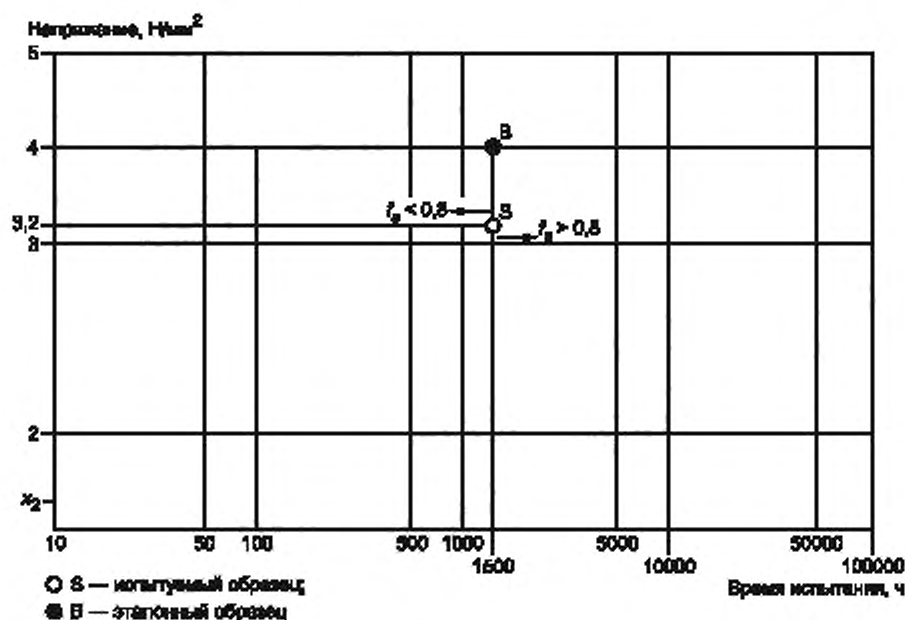
Рисунок 9 — Упрощенный метод подтверждения требуемого коэффициента сварного шва при испытаниях на ползучесть при растяжении
