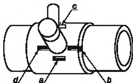
Рисунок Б.3 — Отбор образцов (от а до d) в случае седелок для испытаний на сдвиг со скручиванием: вручную, механизированным методом и радиальным расслаиванием
