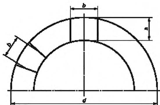
Рисунок 11 — Способы вырезания образцов из трубы
