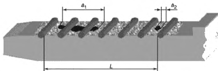
Рисунок А.1 — Длина зоны соединения L и примеры дефектов для образцов соединений, выполненных муфтовой сваркой с закладными нагревателями (ЗН)
