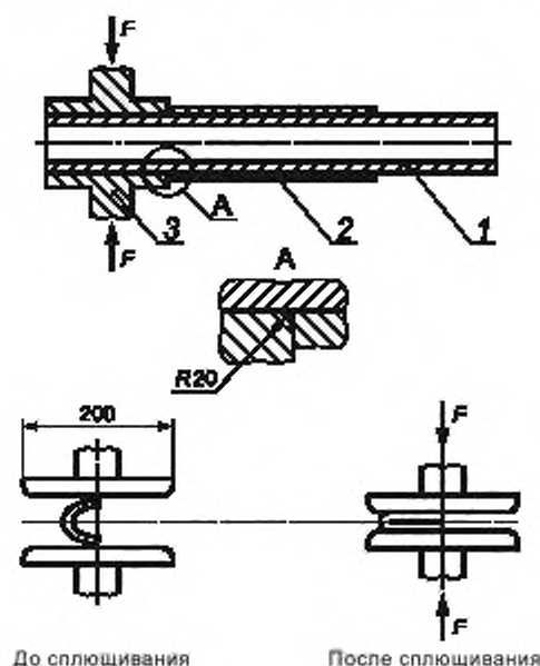
Рисунок 16 — Расположение образцов между плитами испытательной машины
