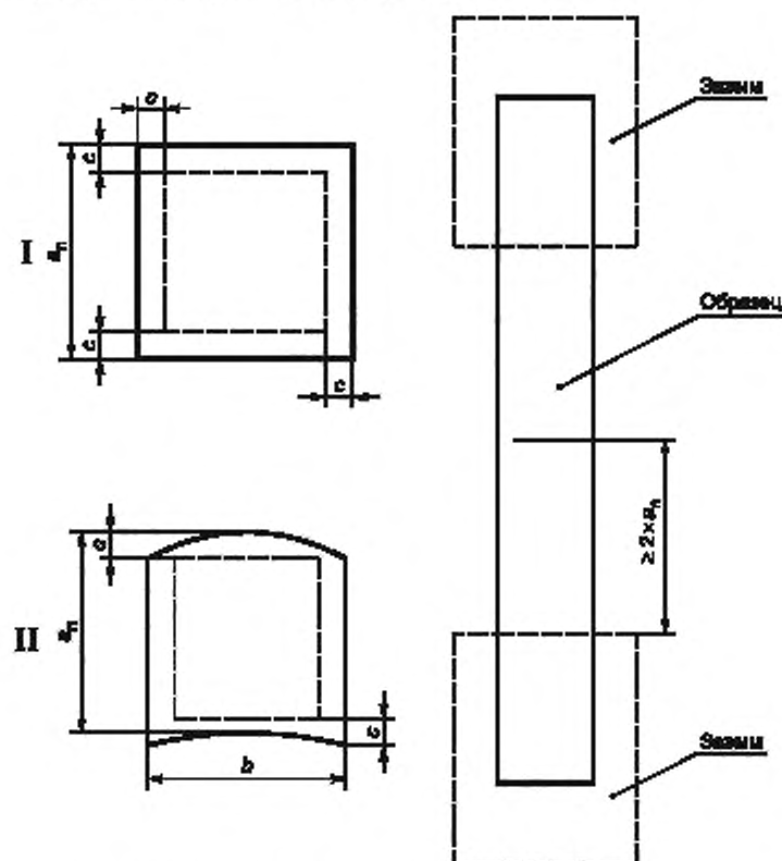
Рисунок Г.1 — Образцы для испытаний
