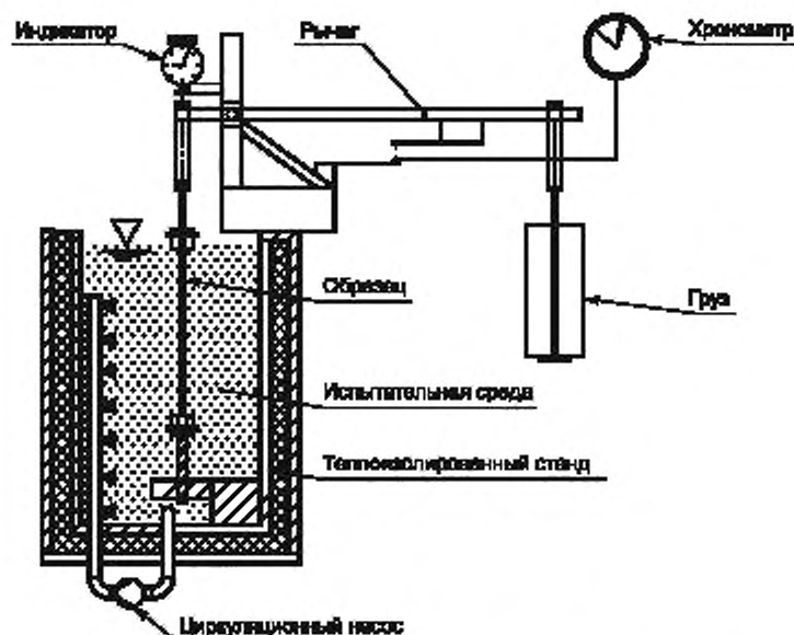
Рисунок 5 — Стенд для испытаний на ползучесть при растяжении
