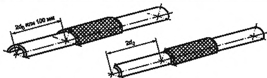
Рисунок 15 — Подготовка испытываемых образцов
