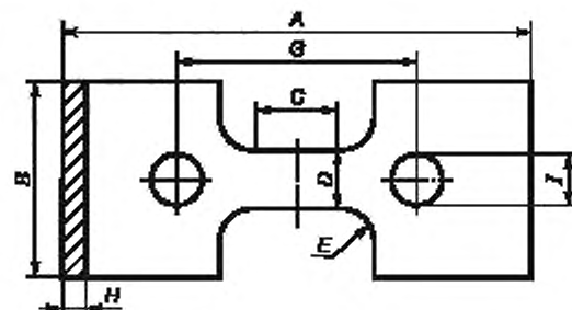
Рисунок 4 — Испытуемый образец, тип 3
