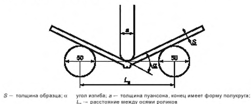
Рисунок 10 — Схема нагружения
