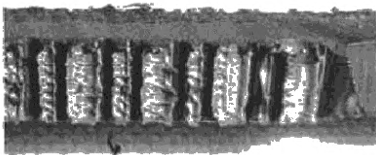
Рисунок Б.7 — Образец ПЭ с пластической поверхностью разрушения
