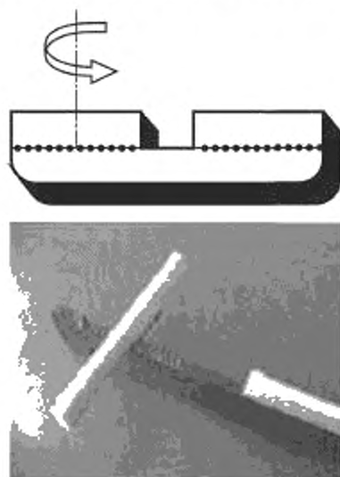
Рисунок Б.4 — Сдвиг кручением вручную
