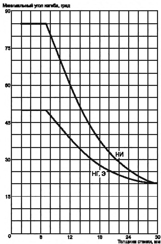
Рисунок В.2 — Минимальный угол загиба для ПП-В, ПП-Г и электропроводящего ПЭ в зависимости от толщины для разных методов сварки (верхняя кривая — для сварки нагретым инструментом встык, нижняя — для пучковой газовой сварки и экструзионной сварки)
