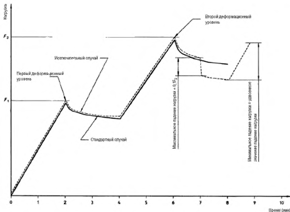
Рисунок 1 – Схематичная диаграмма нагрузки в зависимости от времени
