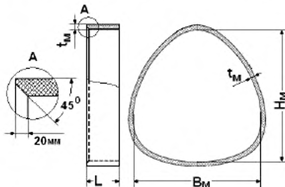
B_M — ширина соединительной муфты по внутренней поверхности стенки; H_M — высота соединительной муфты по внутренней поверхности стенки; L — длина соединительной муфты; t_M — толщина стенки соединительной муфты
