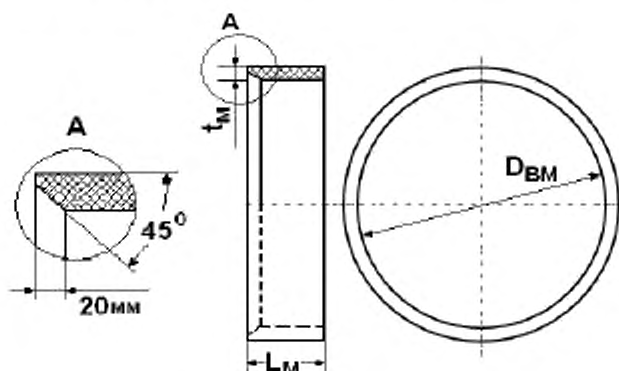
L_M — длина соединительной муфты; t_M — толщина стенки соединительной муфты; D_{BM} — внутренний диаметр соединительной муфты
