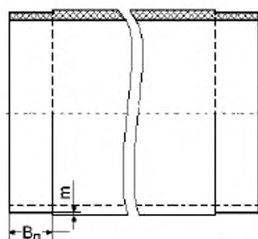
B_{\text{п}} — ширина шлифования под муфту; t — глубина шлифования под муфту
