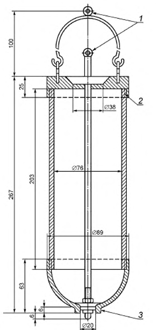
1 — петля для фиксации цели; 2 — резьба; 3 — четыре выступа
