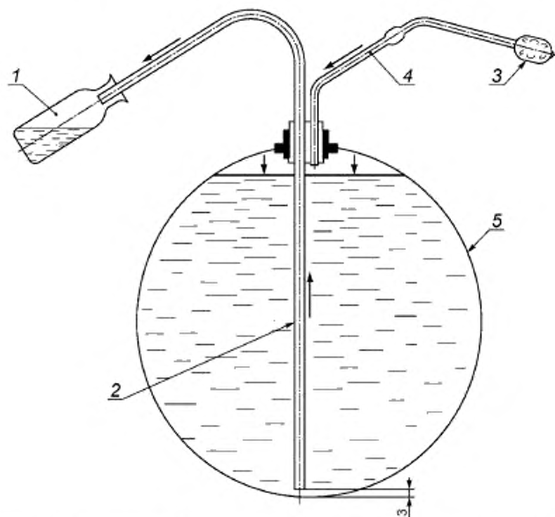
1 — бутылка для проб; 2 — стеклянная трубка внутренним диаметром 13 мм; 3 — нагнетатель воздуха; 4 — металлическая трубка внутренним диаметром 5 мм; 5 — бочка
