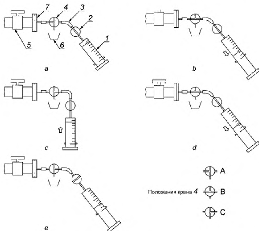
а — промывание; б — смазывание и промывание шприца; в — опорожнение шприца; г — отбор пробы; д — отсоединение шприца; 1 — шприц; 2 — запорный кран; 3 — гибкая соединительная трубка; 4 — трехходовый кран; 5 — пробоотборный кран оборудования; 6 — емкость для отходов; 7 — глухой фланец
