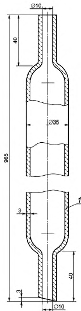
1 — стеклянная трубка, зауженная с обоих концов
