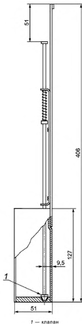
Рисунок 2 — Поверхностный пробоотборник
