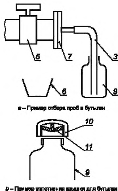
3 — гибкая соединительная трубка; 5 — пробоотборный кран оборудования; 6 — емкость для отходов; 7 — глухой фланец; 9 — бутылка; 10 — твердая пластиковая резьбовая крышка; 11 — мягкое коническое уплотнение из полиэтилена
