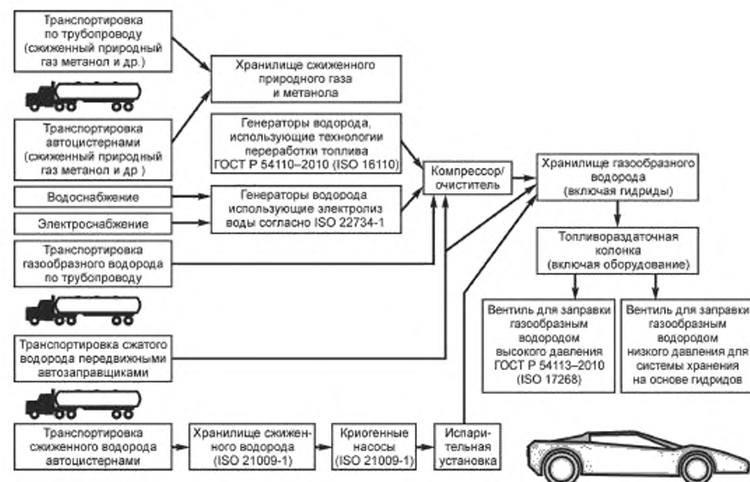
Рисунок 1 — Газообразный водород — заправочная станция
