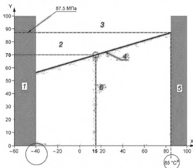
X -- температура ( ^{\circ}\text{C} ); Y -- давление (МПа); 1 -- уровень избыточного охлаждения; 2 -- зона избыточной заправки; 3 -- уровень избыточного давления; 4 -- уровень полной заправки; 5 -- уровень избыточного перегрева; 6 -- рабочая зона; \square -- ограничение заправки
