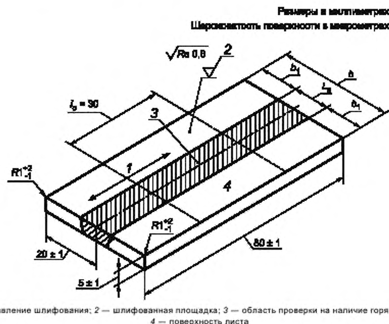
Рисунок 5 — Образец для испытания на продольный изгиб
