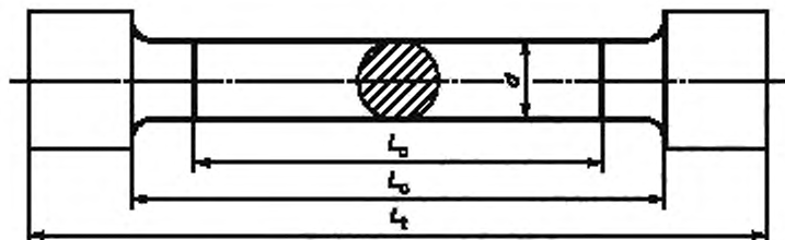
Рисунок 3 — Образец для испытания на растяжение металла шва
